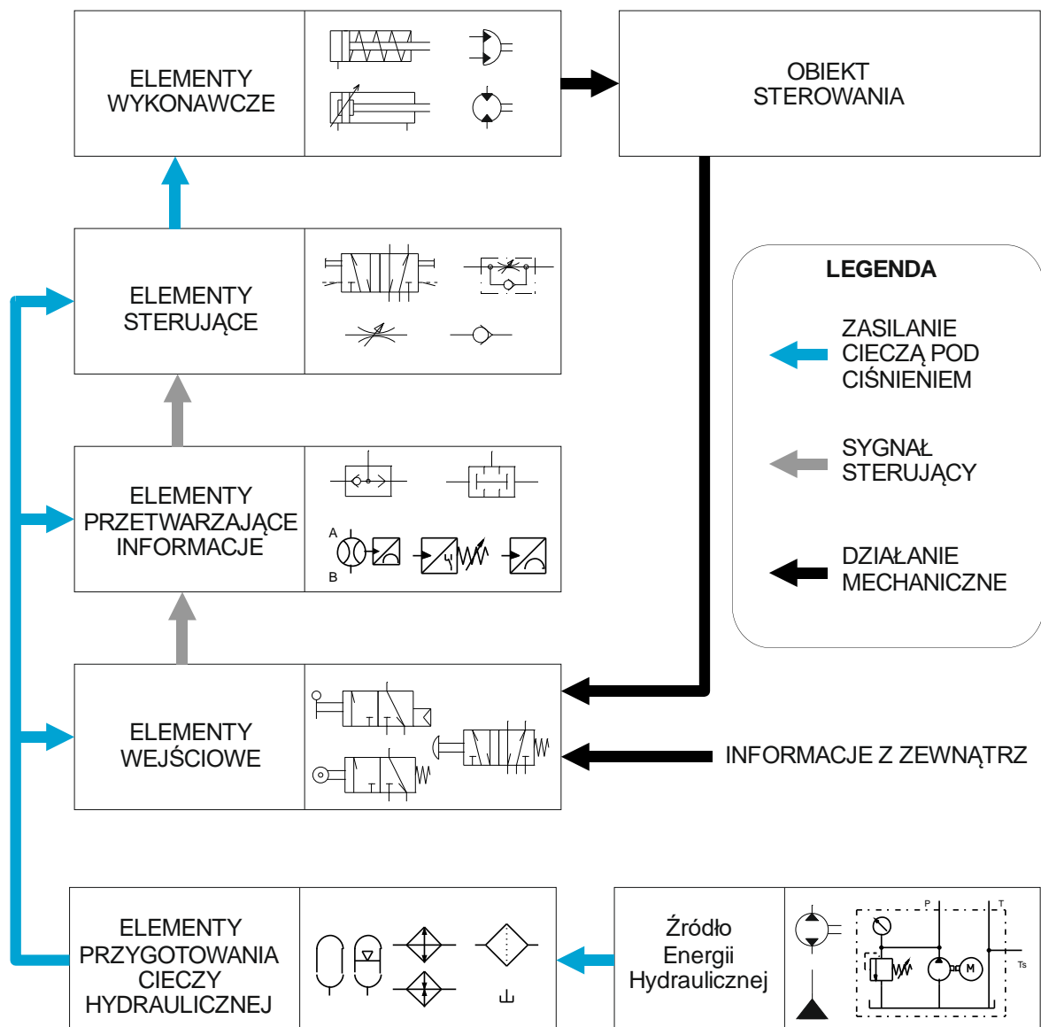
Rys.13.1 Struktura funkcjonalna układu elektrohydraulicznego
