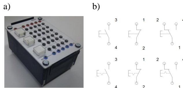
Rys. 13.7. Urządzenie do łączenia sygnałów wejściowych: a) widok urządzenia do łączenia sygnałów wejściowych, b) symbole urządzenia do łączenia sygnałów wejściowych
