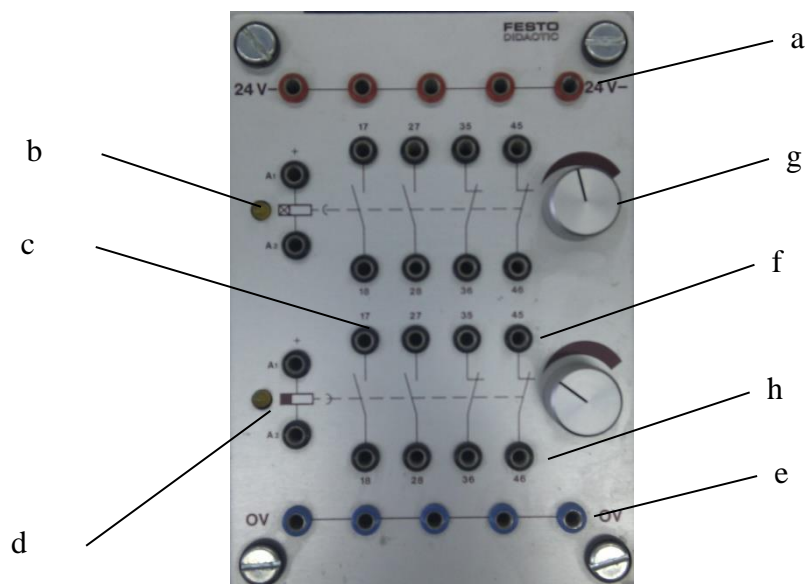
Rys. 13.6. Widok zestawu przełączników czasowych: a) gniazdo zasilania zestawu przełączników czasowych 24 V DC, b) dioda sygnalizująca działanie przełącznika czasowego ze zwłocznym załączaniem, c) gniazdo wejścia styku normalnie otwartego, d) dioda
