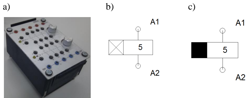
Rys.13.5. Zestaw przełączników czasowych: a) widok zestawu przełączników czasowych, b) symbol przełącznika czasowego ze zwłocznym załączaniem, c) symbol przełącznika czasowego ze zwłocznym zwalnianiem
