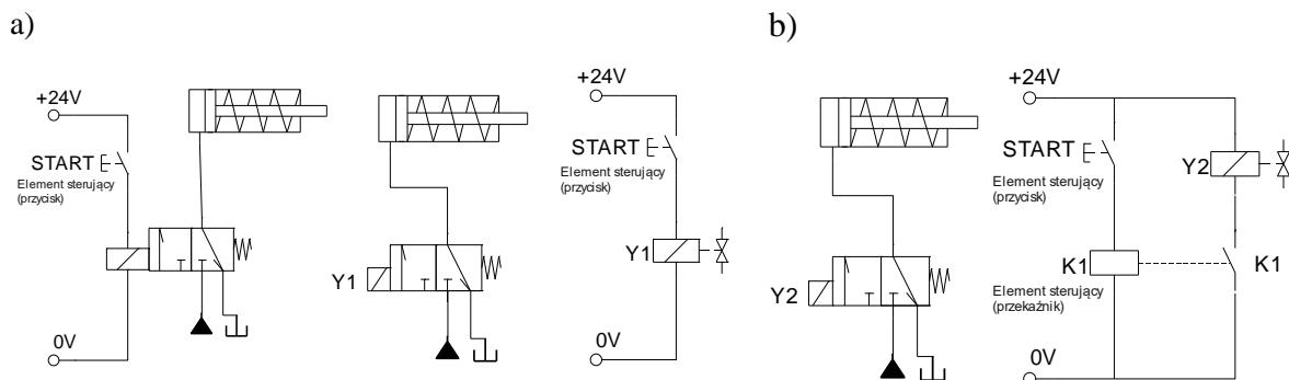
Rys. 13.2. Schemat układu elektrohydraulicznego sterowania siłownika jednostronnego działania z wykorzystaniem zaworu 3/2 sterowanego elektrycznie: a) bezpośrednio, b) pośrednio
